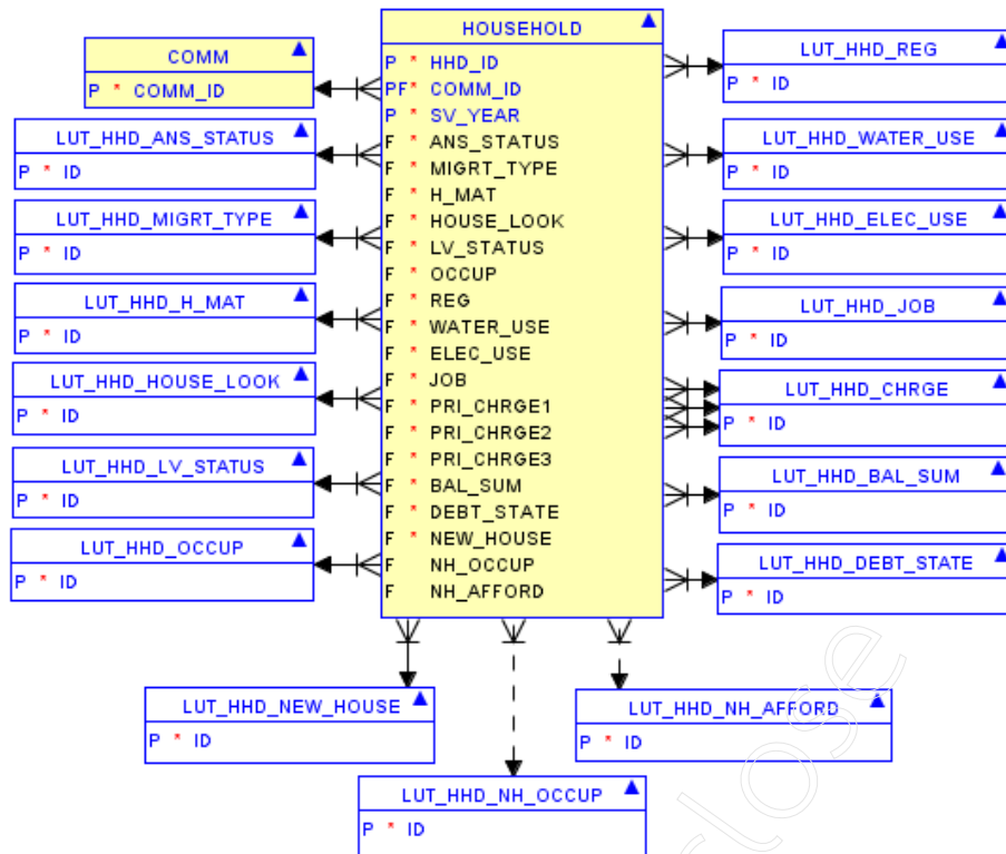
รูปที่ 0-1 แสดง ER Diagram ข้อมูลครัวเรือนชุมชนผู้มีรายได้น้อย
